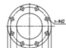
Discharge flange
