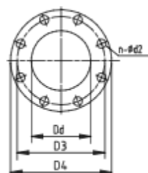
Discharge flange
