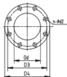
Discharge flange
